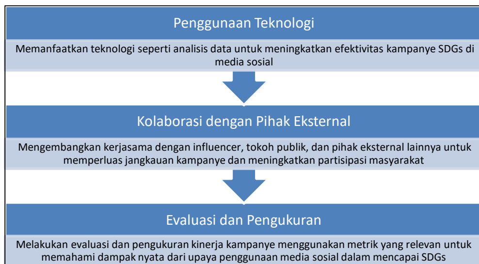
Gambar 2. Langkah-langkah Implementasi
